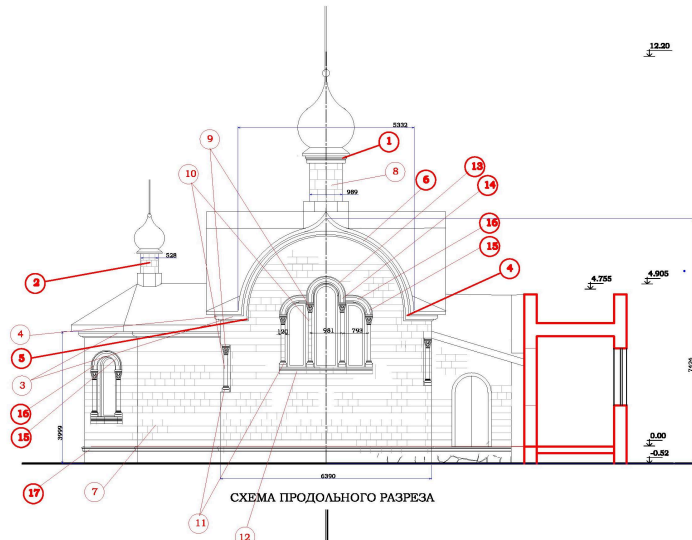
СЕВЕРНЫЙ ФАСАД
