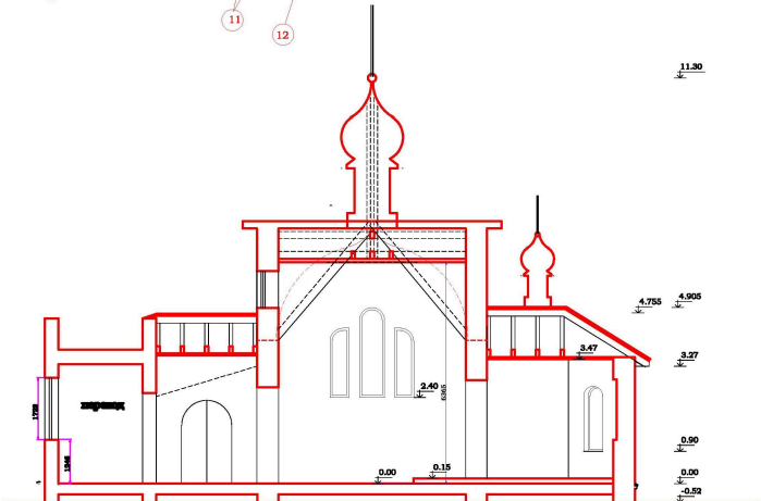
СХЕМА ПРОДОЛЬНОГО РАЗРЕЗА
