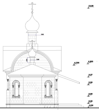
ВОСТОЧНЫЙ ФАСАД
